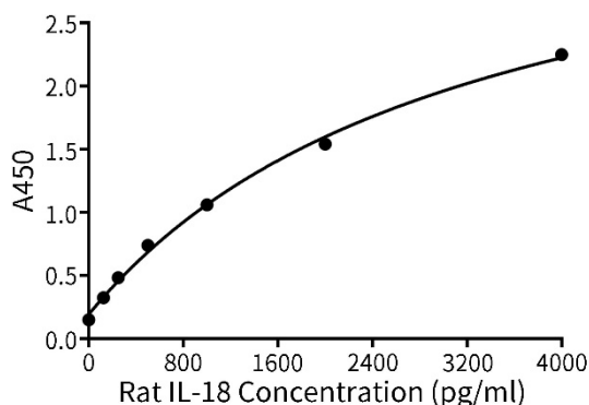
图3. Rat IL-18 ELISA Kit的标准曲线。实测数据会因实验条件、检测仪器等的不同而存在差异，图中数据仅供参考。
